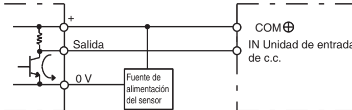
Salida de tensión
