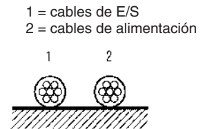
Conductos
