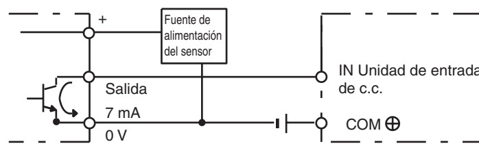
Salida de colector abierto NPN
