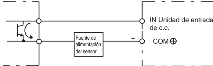
Salida de c.c. de dos hilos
