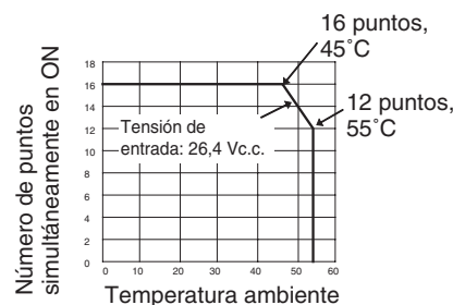
Características térmicas de número de puntos simultáneamente a ON
