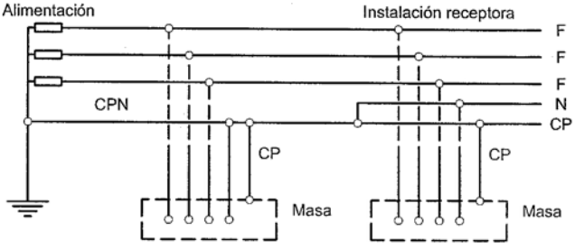
Figura 3. Esquema de distribución tipo TN-C-S
