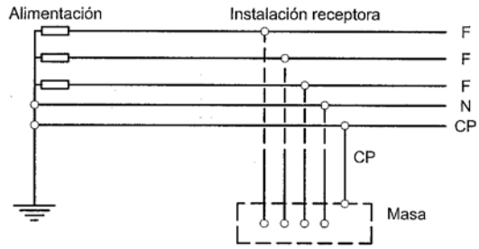
Figura 1. Esquema de distribución tipo TN-S
