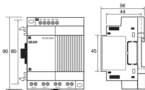
Unidades de expansión de E/S (4 entradas, 4 salidas, 8 E/S)
