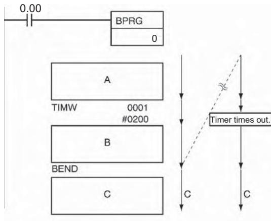
Coding
